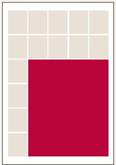
4x4 16 modułów 199,2x240,4 mm
