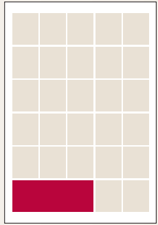
3x1 3 moduły 148,4x57,5 mm
